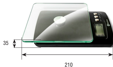
Dimensiones (mm)
